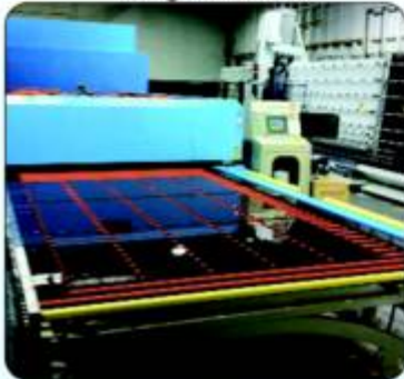
Round Table Top Beveling Edgine
